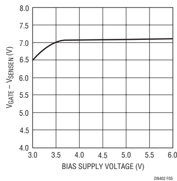
图 5：栅极驱动电压与偏置电源电压的关系
